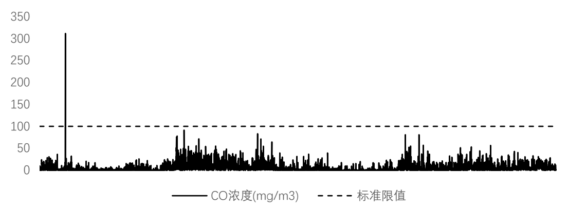
图3-4 一氧化碳排放浓度在线监测统计
