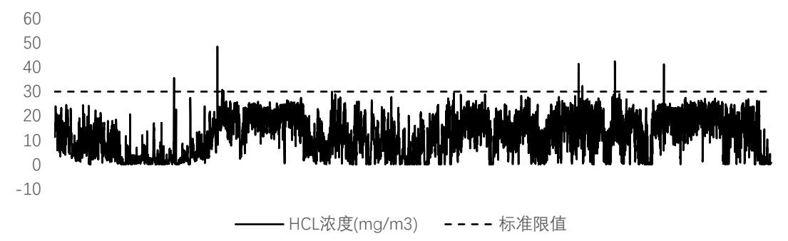
图3-5 氯化氢排放浓度在线监测统计
