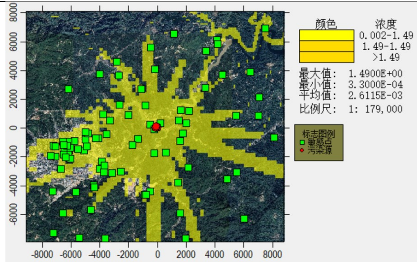
图6-17 硫化氢小时浓度分布图
