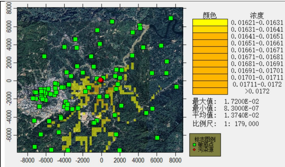
图6-2 PM2.5 日均保证率浓度分布图
