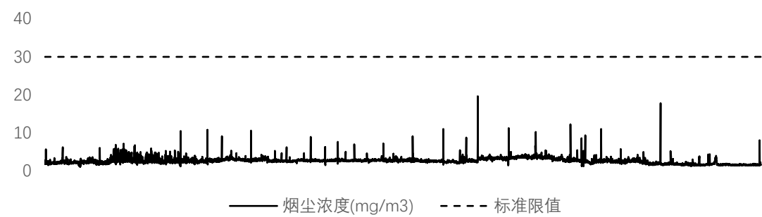
图3-1 烟尘排放浓度在线监测统计
