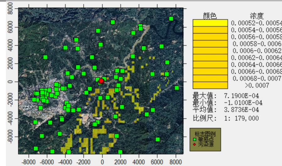
图6-13 镉年均浓度分布图
