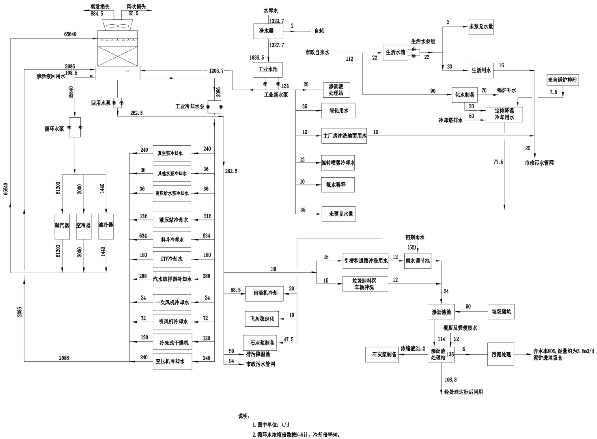
图4-6 水平衡图
