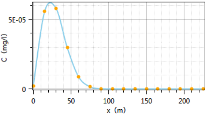
图6-26 非正常状况下污染物 Pb 泄露 100 天污染物扩散结果
