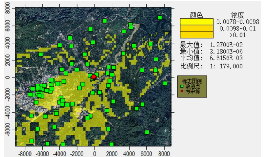
图6-9 氮氧化物年均保证率浓度分布图
