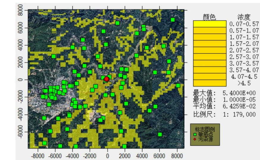
图6-19 氯化氢日均浓度分布图
