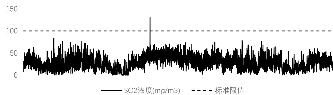
图3-2 二氧化硫排放浓度在线监测统计
