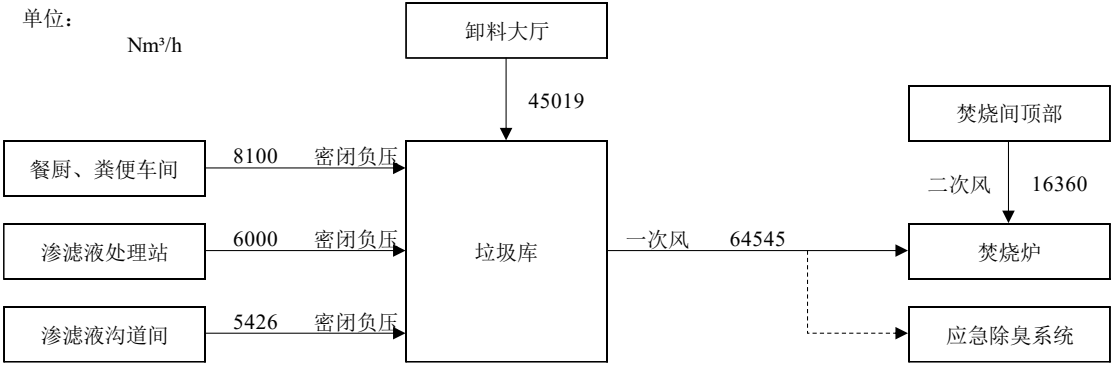
图7-1 臭气系统风量平衡图
