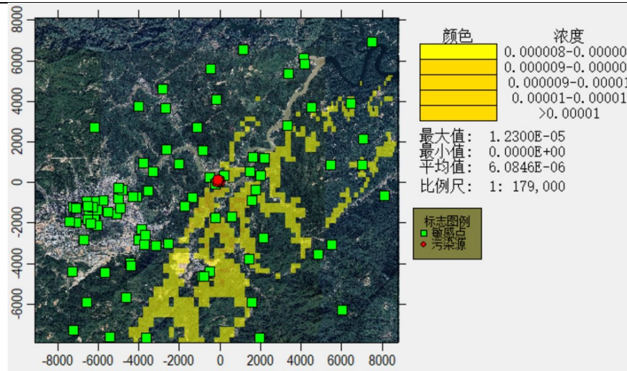
图6-15 二噁英年均浓度分布图
