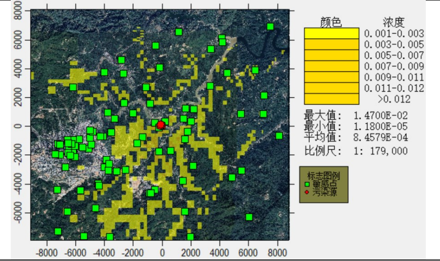
图6-11 一氧化碳日均保证率浓度分布图
